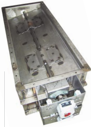
Serranda monopala con movimentazione elettromeccanica DIMENSIONI a richiesta
